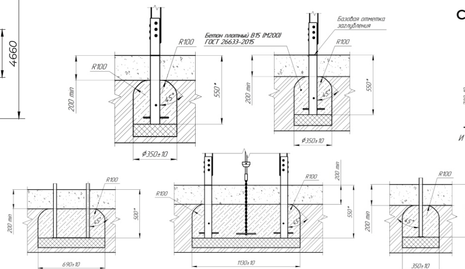
УСТАНОВКА СТОЕК ОБОРУДОВАНИЯ
