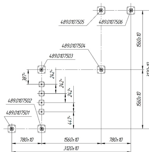
ПЛАН ОБОРУДОВАНИЯ В ОСЯХ
