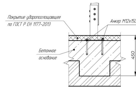
УСТАНОВКА ОБОРУДОВАНИЯ
