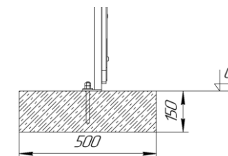
УСТАНОВКА ОБОРУДОВАНИЯ
