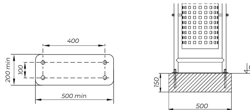
ПЛАН ОБОРУДОВАНИЯ В ОСЯХ
